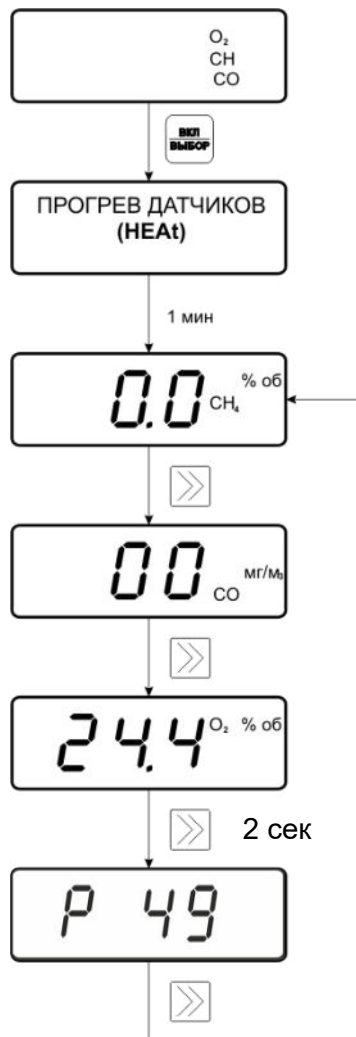
Рисунок 5.1 –Схема режима«РАБОТА»
